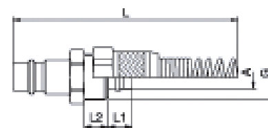
Nippel für Schlauch mit Überwurfmutter und Knickschutzfeder
