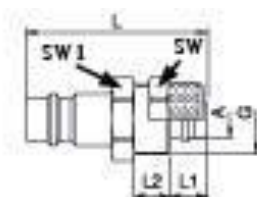
Nippel für Schlauch
