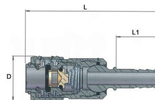
Schlauchtülle, drehbar
