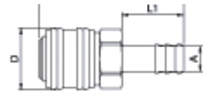
Schlauchtülle
