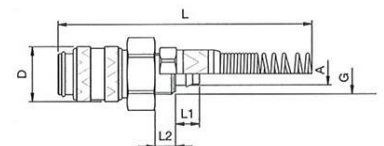
Kupplung mit Überwurfmutter und Knickschutzfeder
