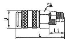
Schlauchanschluss
