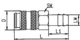
Schlauchtülle
