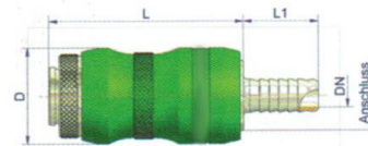
Schlauchanschluss
