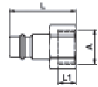
Nippel Innengewinde
