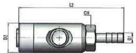
Schlauchanschluss
